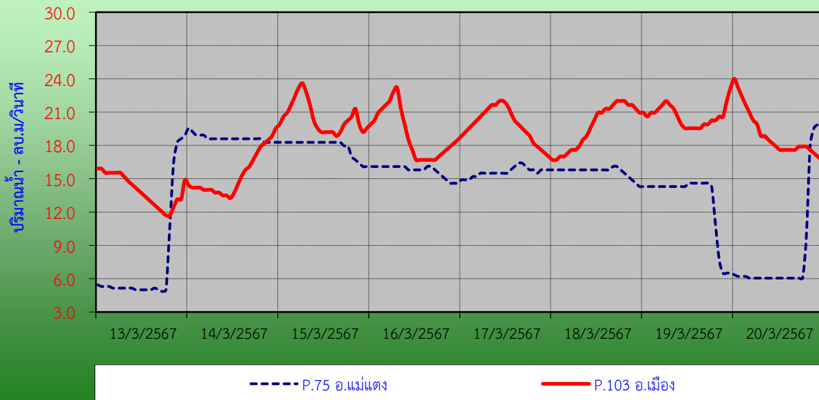
กราฟแสดงปริมาณน้ำปิ้งรายชั่วโมงรอบวันที่ 11/2567 ที่สถานีแม่ น้ำปิ้ง ( P.75) บ้านช่อแล อ.แม่แตง และที่สถานีแม่ น้ำปิ้ง (P.103) บ้านป่าข่อยใต้ อ.เมือง จ.เชียงใหม่
